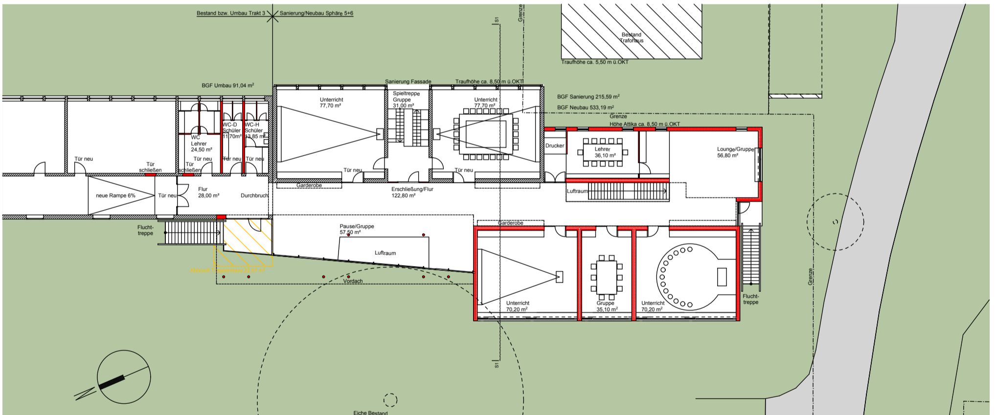
GRUNDRISS OBERGESCHOSS
