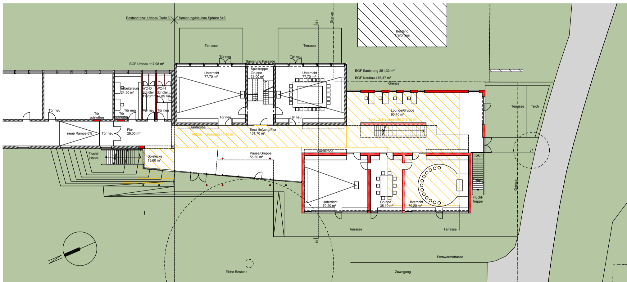
GRUNDRISS ERDGESCHOSS
